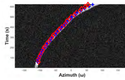
(d) Proposed: SNR = -8 dB
